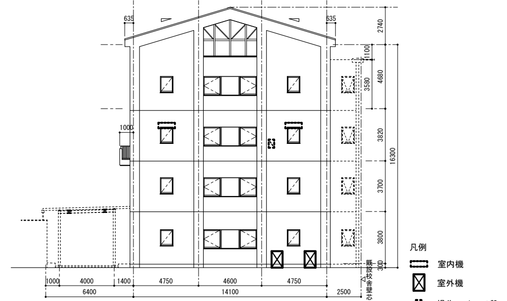
北立面图 S=1/200
