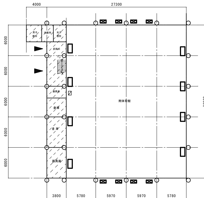
南体育館 1階平面図 S:1/300
