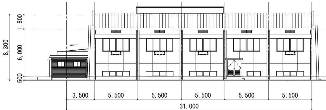
東立面図 S=1/200
