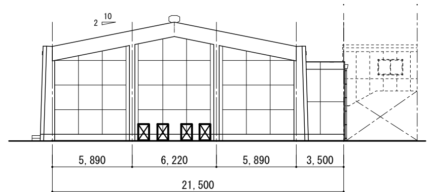
北立面図 S=1/200
