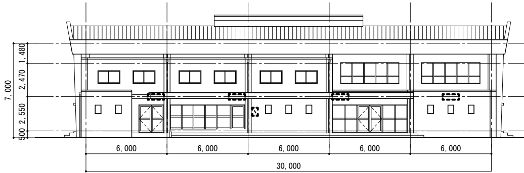
西立面图 S=1/200
