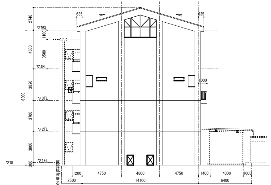
南立面图 S=1/200
