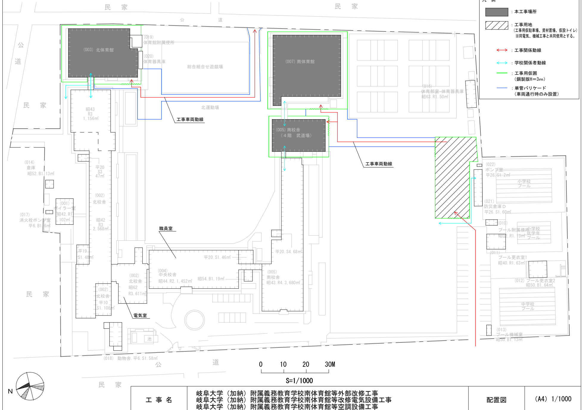
別図①【校内工事車両通行時】（夏休み期間（R8.7.18～8.25）及び、R8.8.26からの土日祝日）
