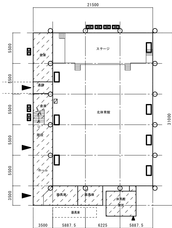
北体育館 1階平面図 S:1/300
