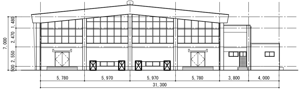
北立面图 S=1/200
