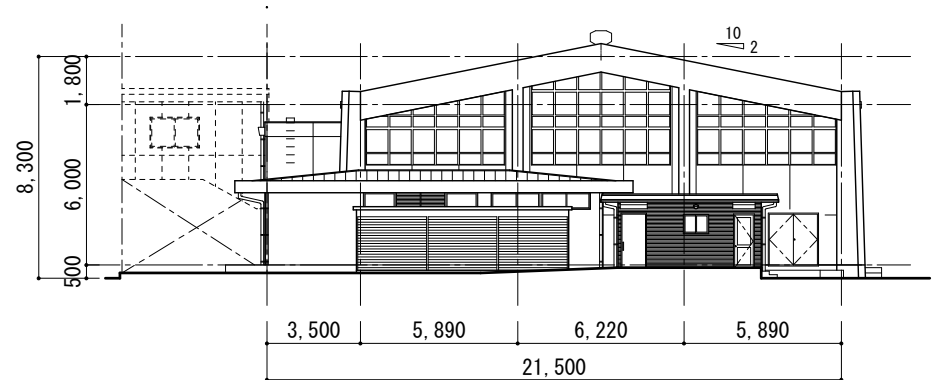
南立面図 S=1/200
