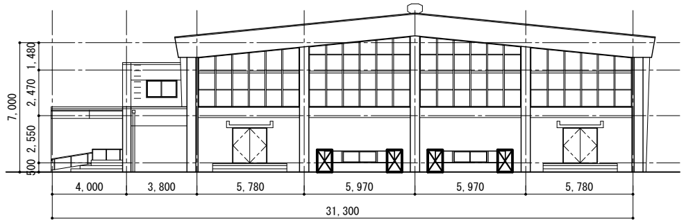
南立面图 S=1/200
