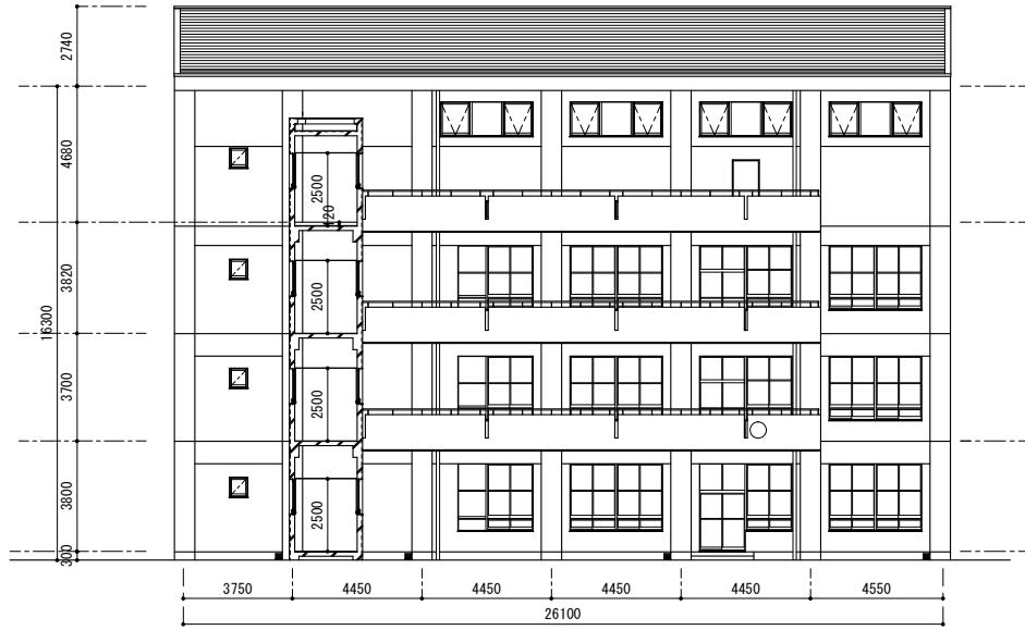
西立面图 S=1/200
