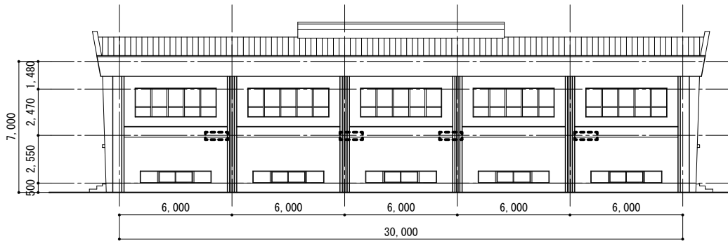
東立面图 S=1/200
