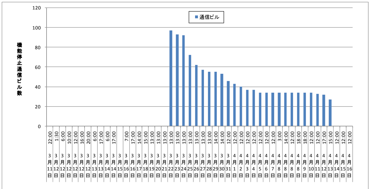
図 1 1 機能停止通信ビル数の推移 (NTT 東日本)
