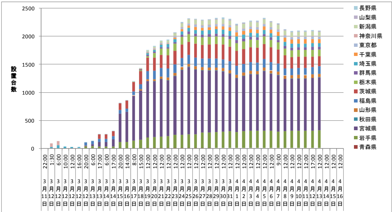
図 1 3 無料公衆電話等の設置台数の推移 (NTT 東日本)
