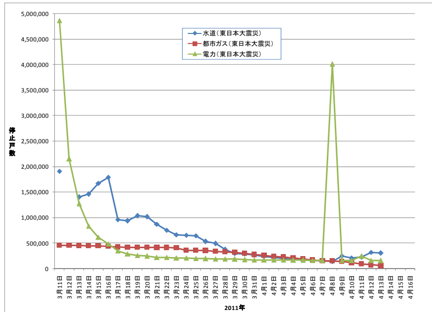
図18 東日本大震災における水道・都市ガス・電力の停止戸数の解消過程 (電力については東北電力管内のみ)
