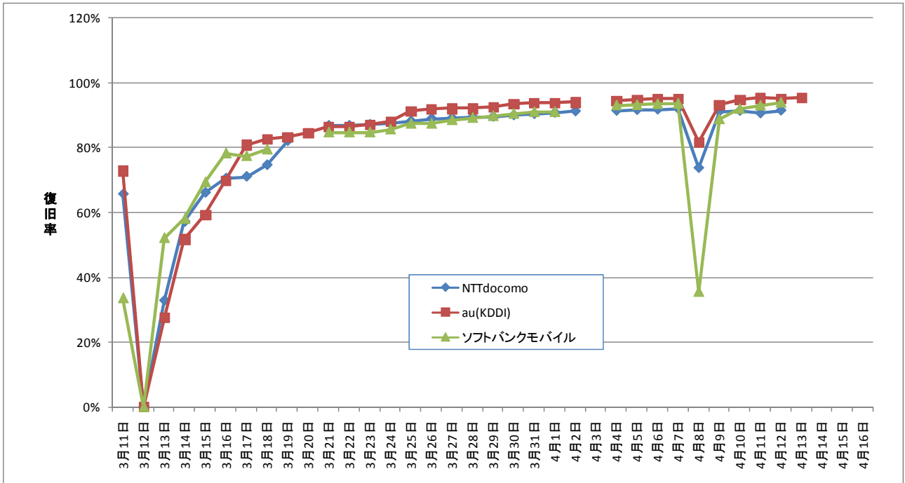
図 1 6 「復旧率 = (最大停止局数 - 停止局数) / 最大停止局」の推移 (3月12日停止局数ベース)
