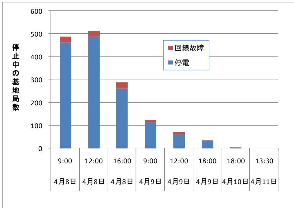
図 1 7 4 月 7 日 23 時 32 分の余震による停止基地局数の原因別内訳 (KDDI)
