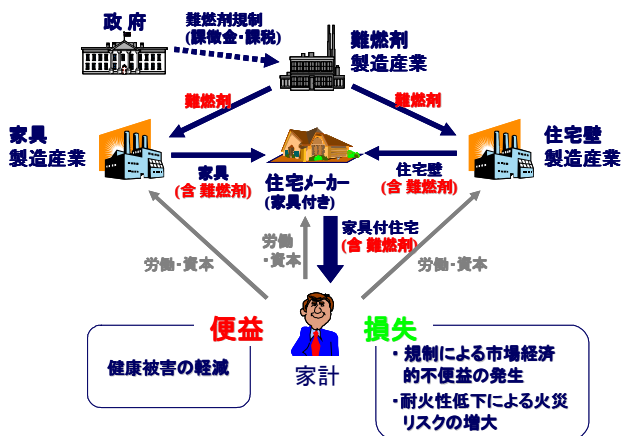
図-1 難燃剤規制策実施の影響
