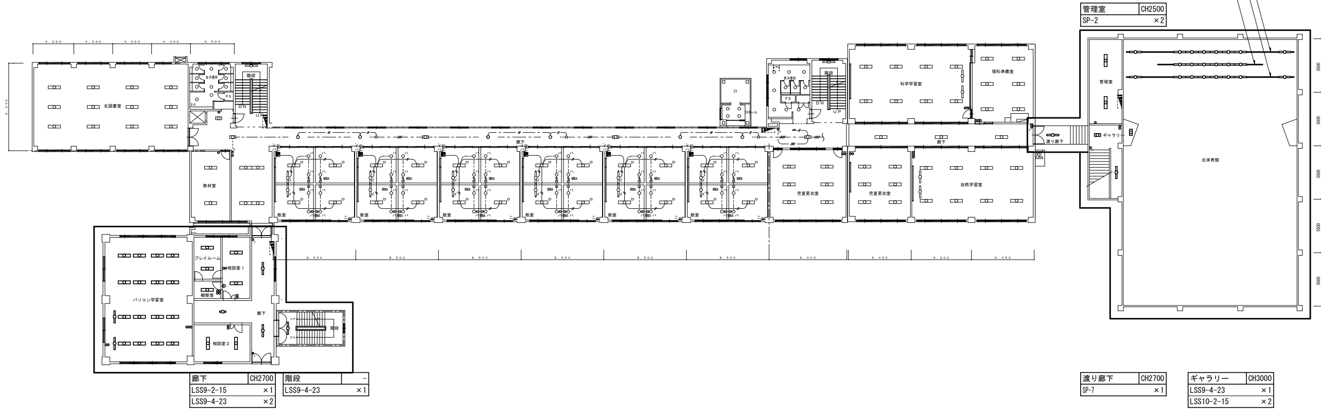
義務教育学校 北校舎・北体育館 2階 電灯設備(改修後) S=1/400
