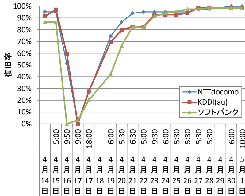
図 5.4 「復旧率 = (最大停止局数 - 停止局数) / 最大停止局」の推移 (各社の最大停止局数で基準化)
