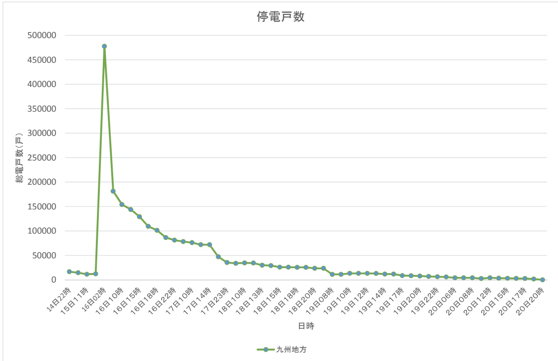
図 2.1(a) 停電戸数の解消過程（九州電力全体，ピークは4月16日2時）
