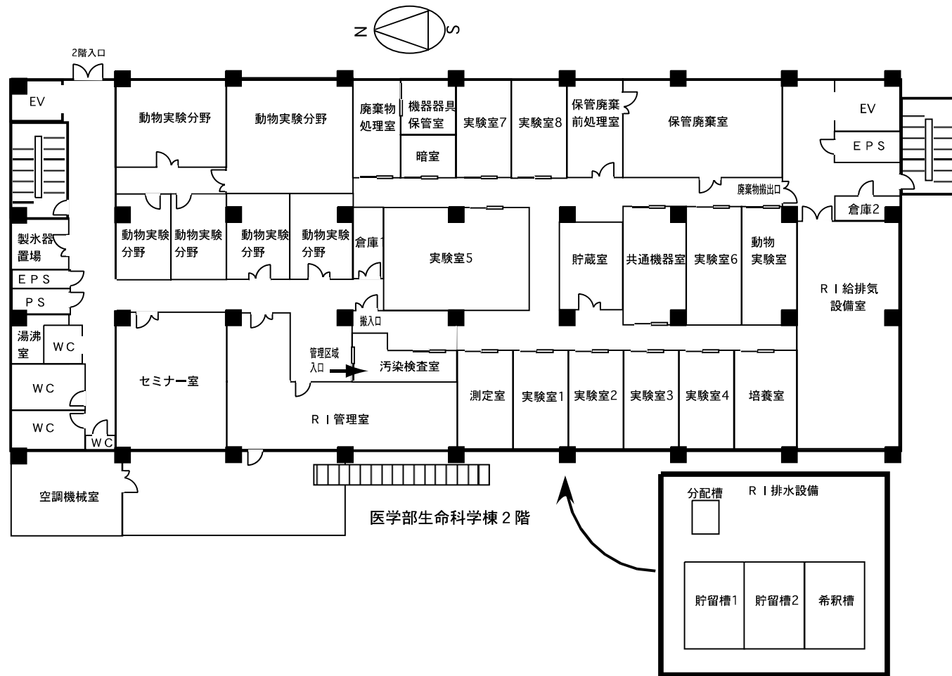
平面詳細図
