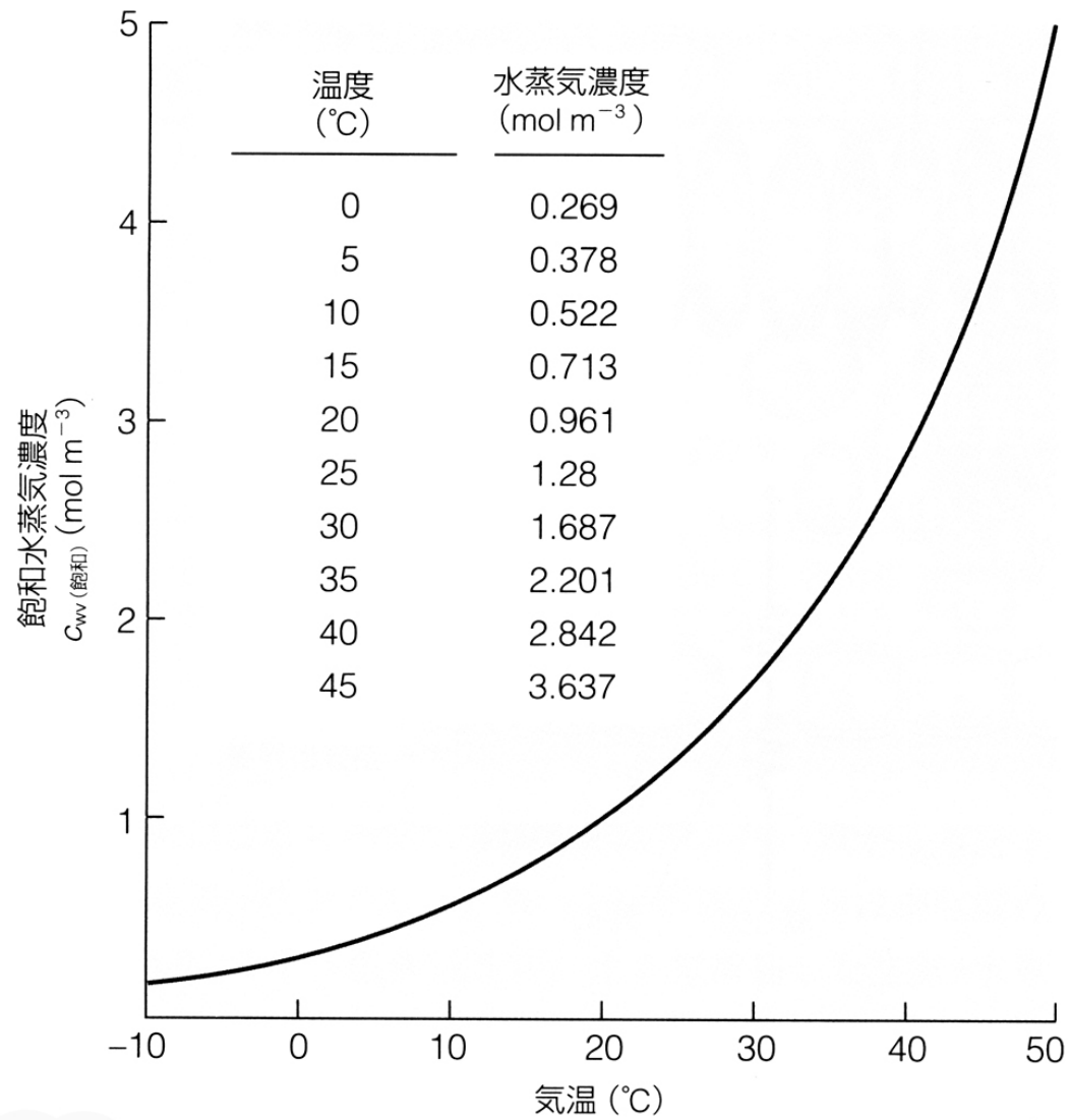
飽和水蒸気濃度と気温との関係
